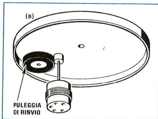
(B) TRASMISSIONE CON PULEGGIA DI RINVIO: semplice ed affidabile, questo metodo di trasmissione ha fornito per molti anni l'elevata coppia di avviamento necessaria per il cambiadischi. Tuttavia, il suo isolamento fra il piatto girevole ed il motore è basso.
