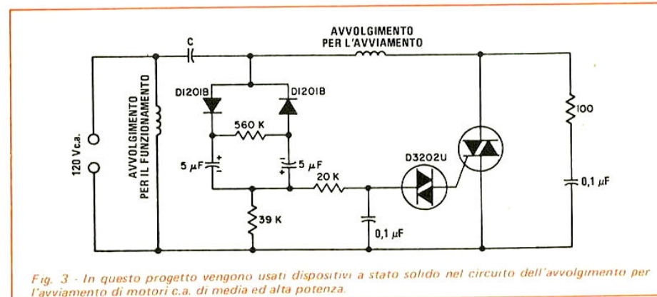
Fig. 2 - Tipico circuito attenuatore di luci con triac che può anche essere usato per il controllo di motori. I valori dei componenti dipendono dai tipi di dispositivi impiegati e dall'applicazione desiderata.
