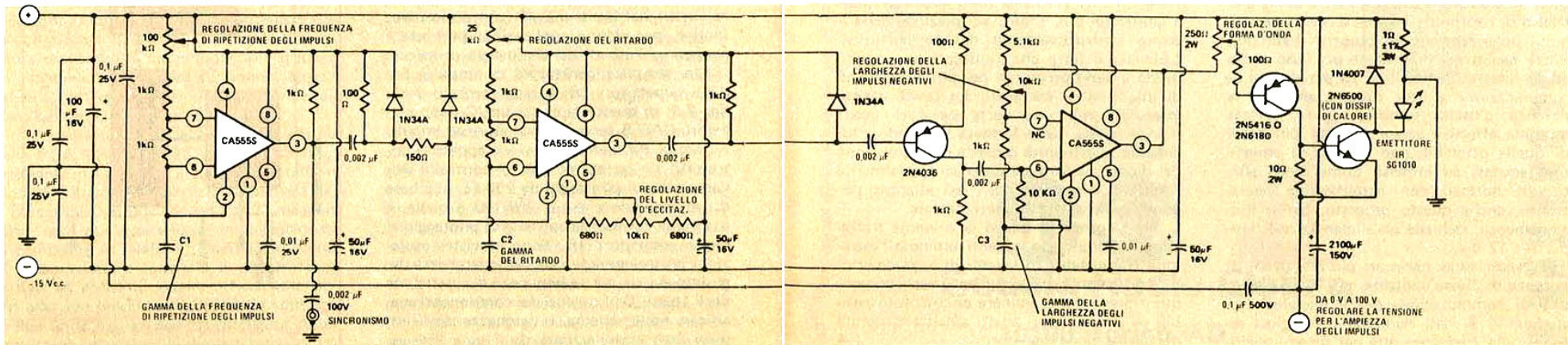
Fig. 3 - Schema di circuito ad alte prestazioni per l'eccitazione ad impulsi di emettitori infrarossi.
