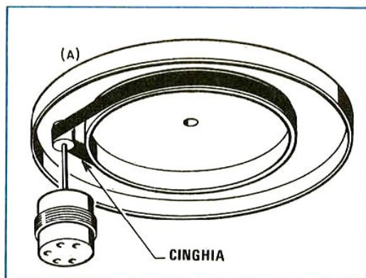
(A) TRASMISSIONE A CINGHIA: la flessibile cinghia "assorbe" la maggior parte delle vibrazioni trasmesse dal motore e le variazioni di velocità, per cui un giradischi con tale tipo di trasmissione, se ben progettato, offre di solito un rumble ed un flutter estremamente ridotti.
