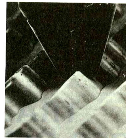
Fig. 3 - La speciale puntina della Stanton segue le creste degli stampi metallici grazie alla sua punta sdoppiata.
